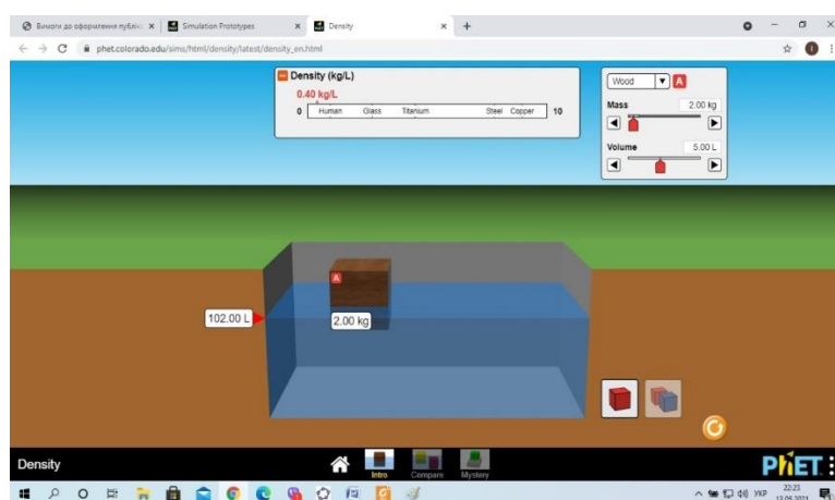
Рис. 4. Архімедова сила.
